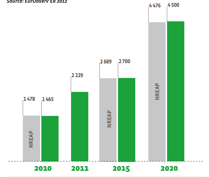
Tendance actuelle de la consommation de chaleur biogaz par rapport à la feuille de route des Plans d'action nationaux énergies renouvelables (en ktep) Comparison of the current trend of biogas heat consumption against the NREAP (National Renewable Energy Action Plans) roadmap (ktep)
